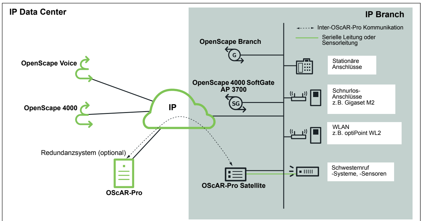
OScAR-Pro Einsatzübersicht
